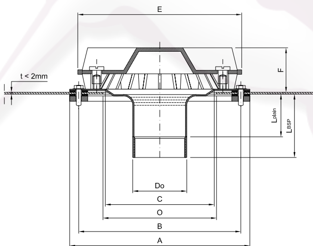
Montaje para canalón Tipo 1 ( t < 2\text{mm} )
