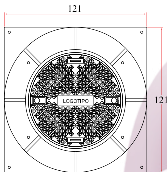
Vista superior
