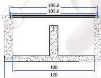
DETALLE DE INSTALACIÓN
