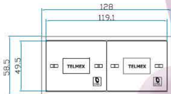
VISTA SUPERIOR
