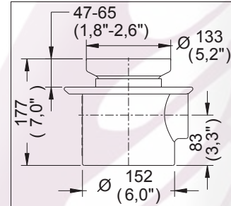
Acot.mm.(pulg)
