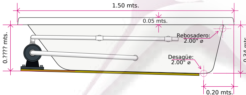
Vista lateral
