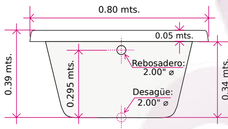
Vista desagüe
