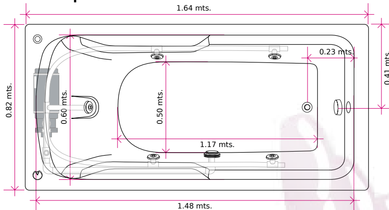
Vista superior
