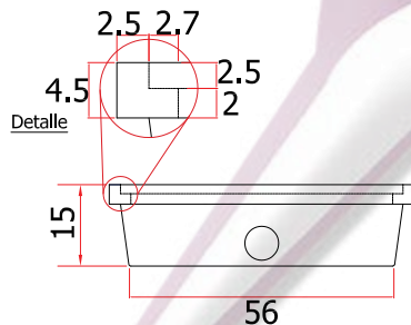
Vista frontal en corte
