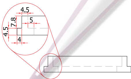
Vista frontal en corte
