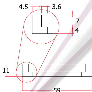
Vista frontal en corte
