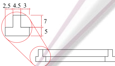
Vista frontal en corte
